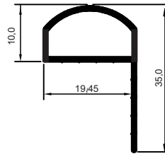
35 mm radüslü tezgha alın profili
