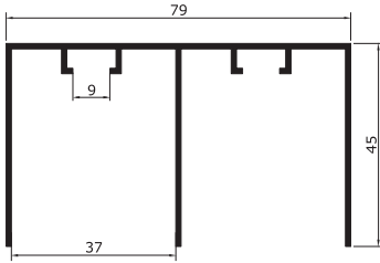
Çiftli Frenli Üst ray
