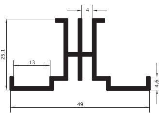
Kanalı çiftli dikme profili
