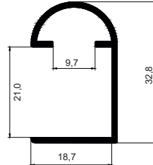
35 mm radüslü tezgha alın profili
