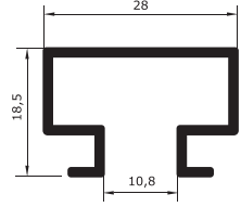
Kanalı tel askılık profili
