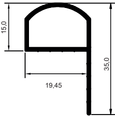
35 mm radüslü tezgha alın profili
