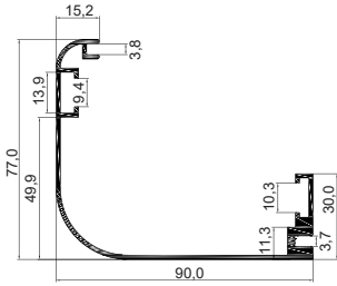
12 - 15 Pervaz profili
